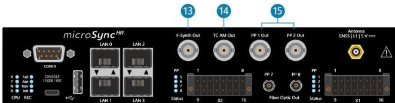
Рисунок 2. Передняя панель Метроном-microSync HR 1xx
